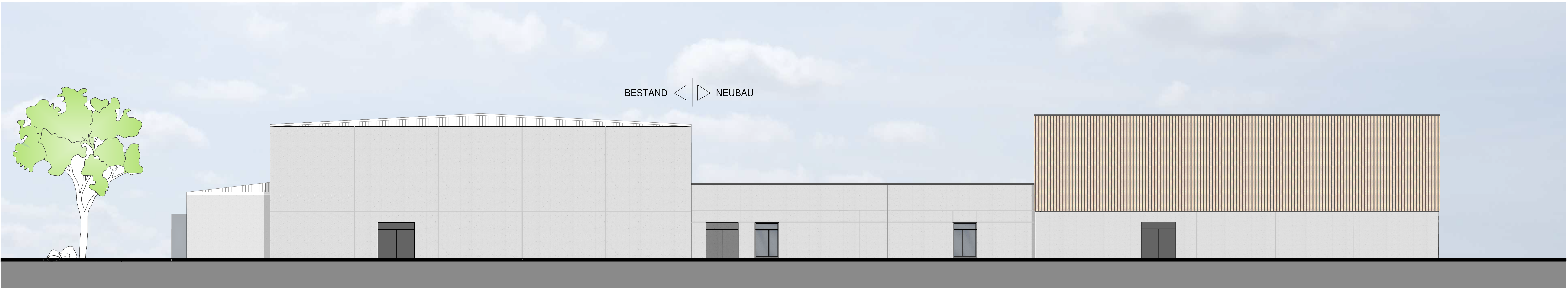
ANSICHT OSTEN
